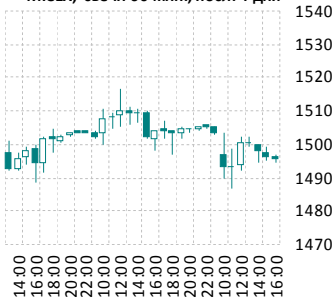
МІСЕХ, свечи 60 мин., посл. 4 дня
