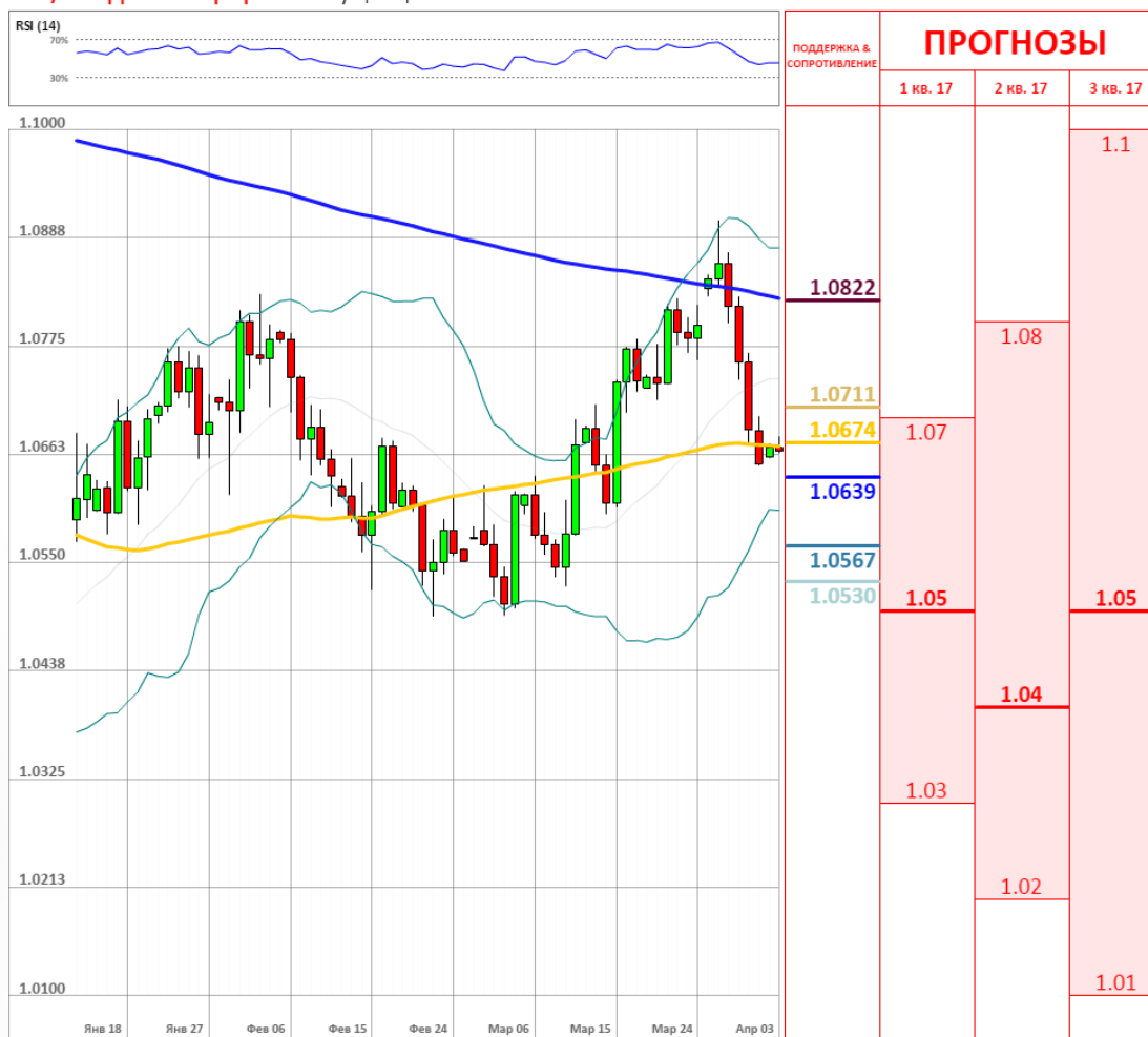
EUR/USD Дневной график Текущая цена 1.0666
